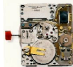
IWC participă la dezvoltarea mașinării cu quartz Beta 21; este primul calibrul de ceas brățară dotat cu o comandă cu quartz (frecvență de oscilare 8192 hertz) - o revoluție în domeniul ceasornicăriei. Foto: © IWC.
