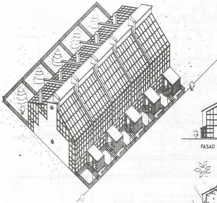
AXONOMETRI
