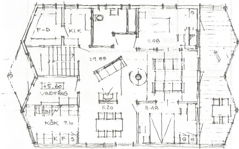
Förslag till enfamiljshus i Vaxholm (skiss), 1987.
